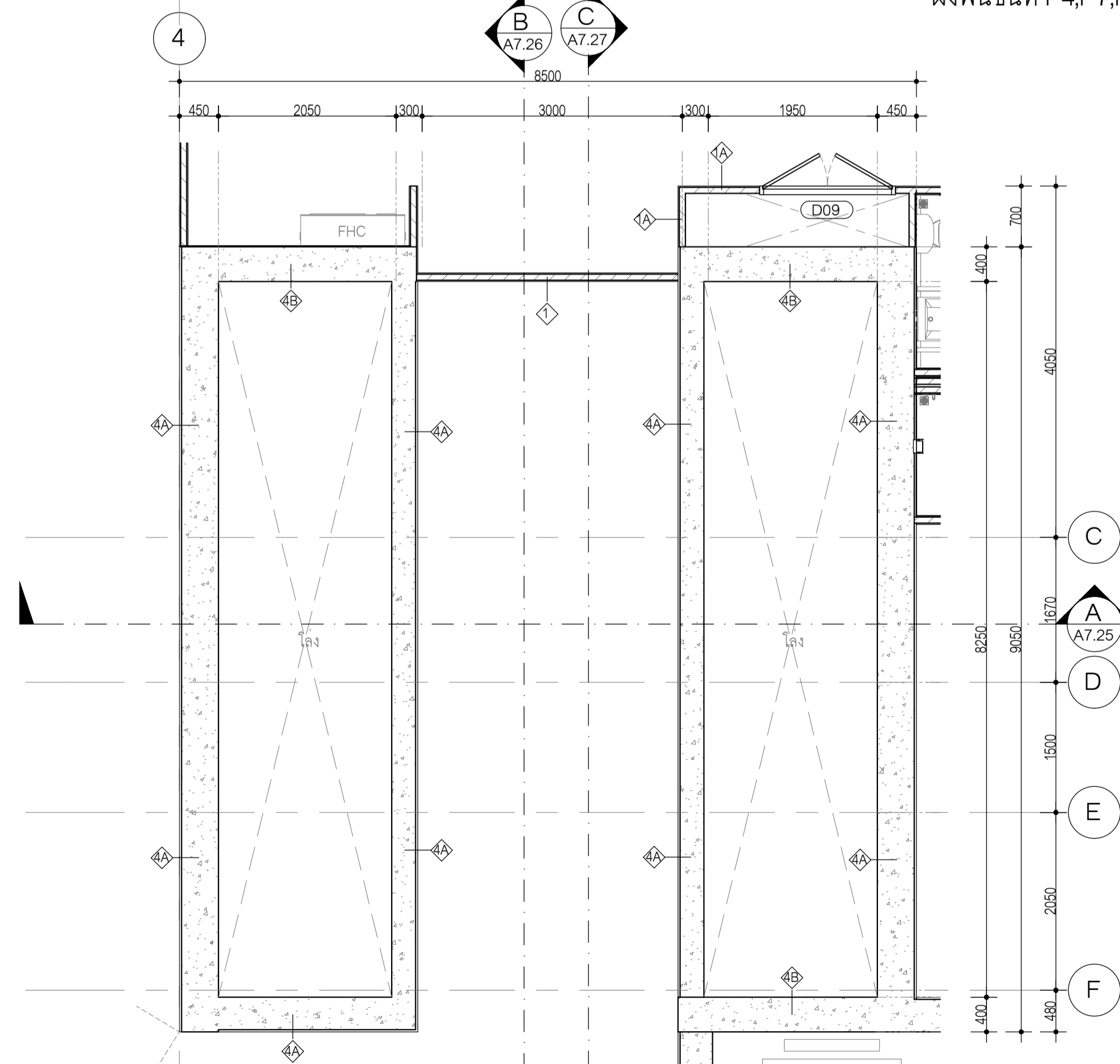
ผังพื้นที่ P2,P3,P5,P6,P8,P9
