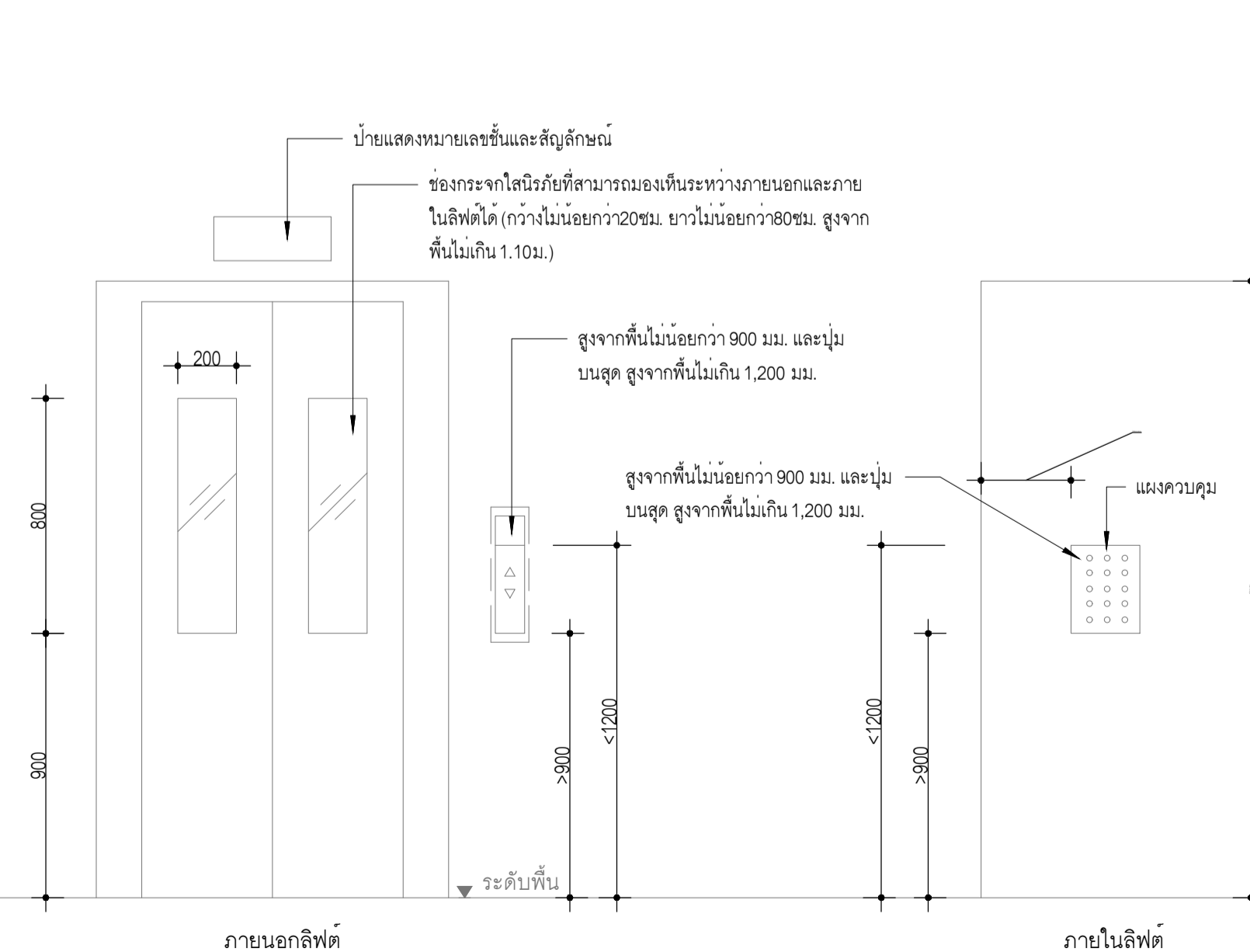
แบบขยายมุมมองหน้าลิฟต์ผู้พิการ
