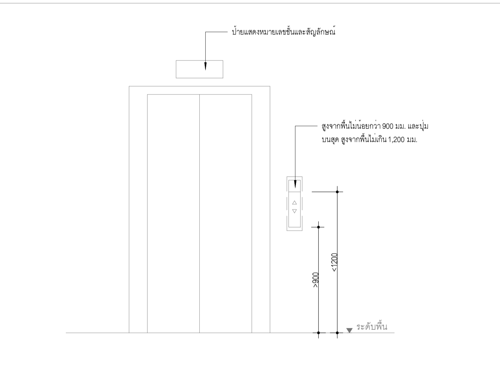
แบบขยายมุมมองหน้าลิฟต์ทั่วไป
