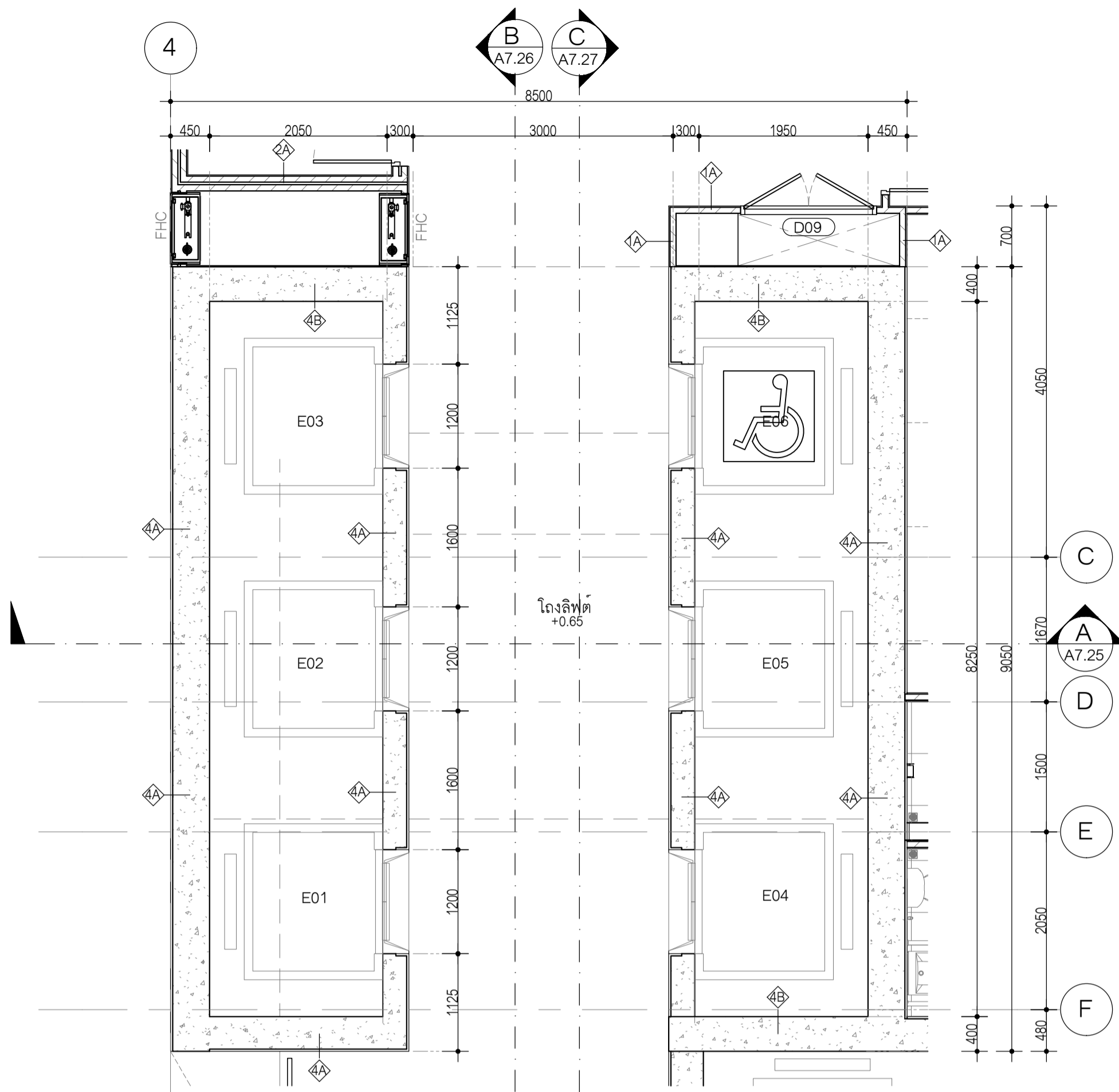
ผังพื้นที่ 1
