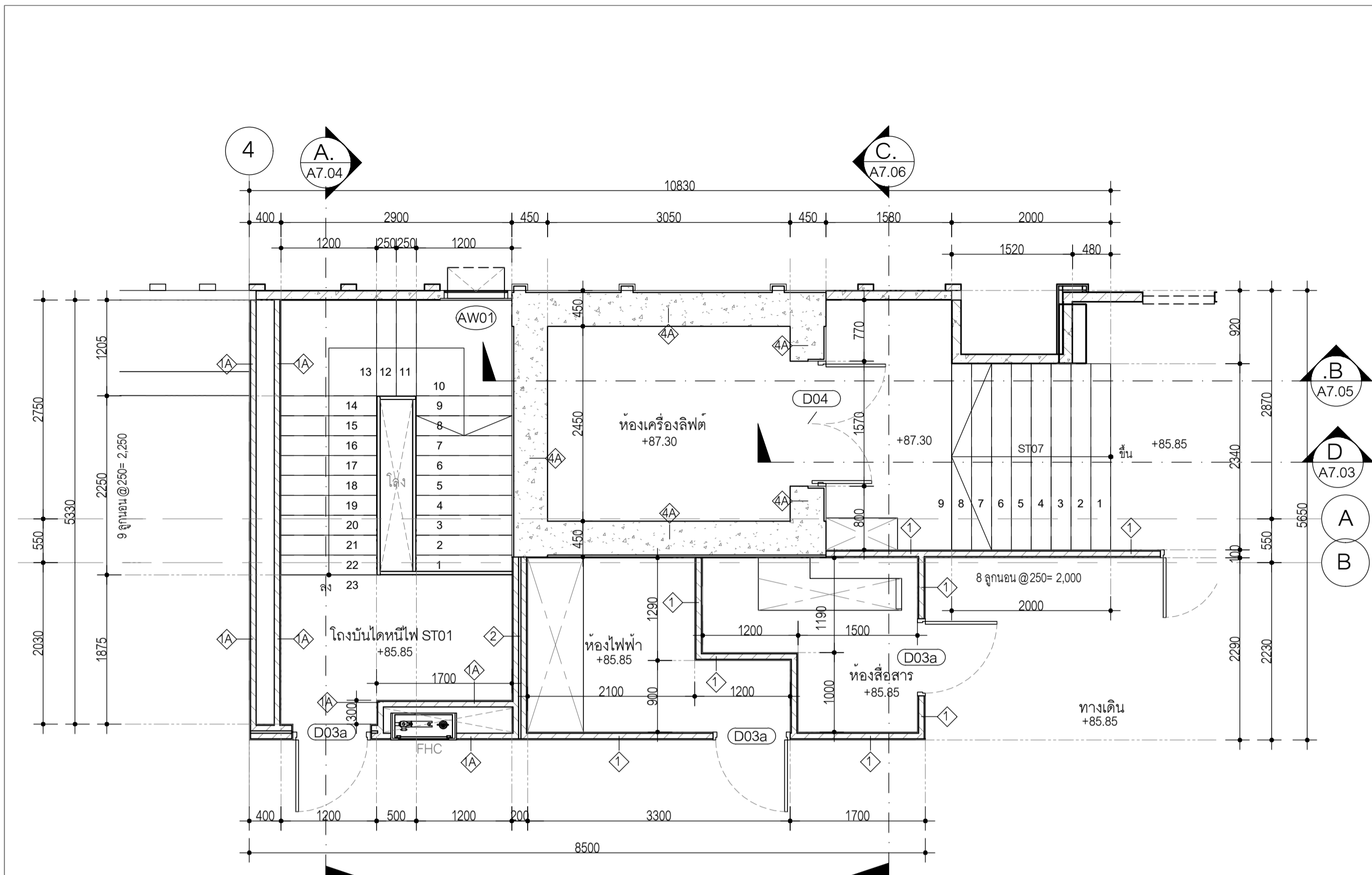
ผังพื้นชั้นหลังคา
