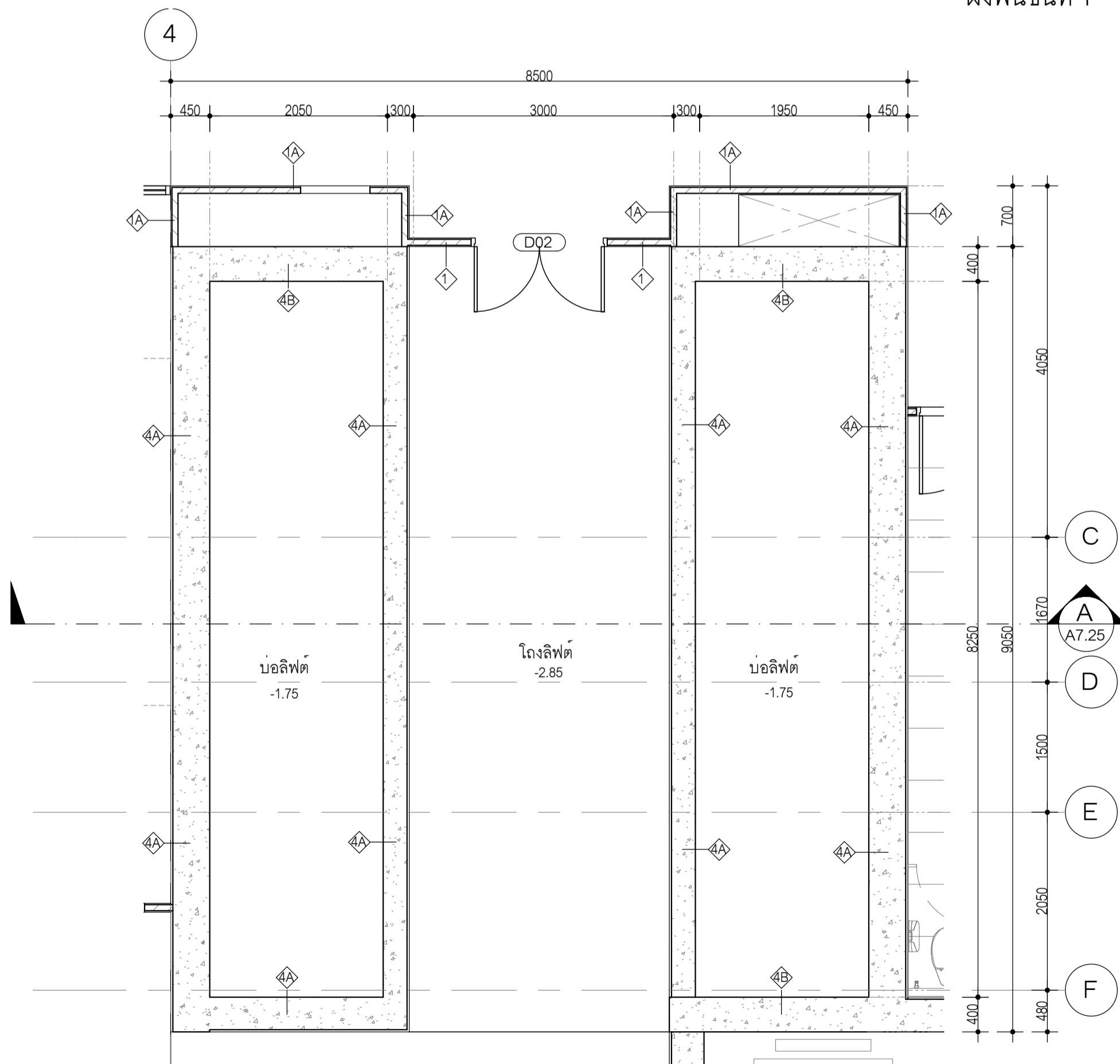
ผังพื้นที่ใต้ดิน B1
