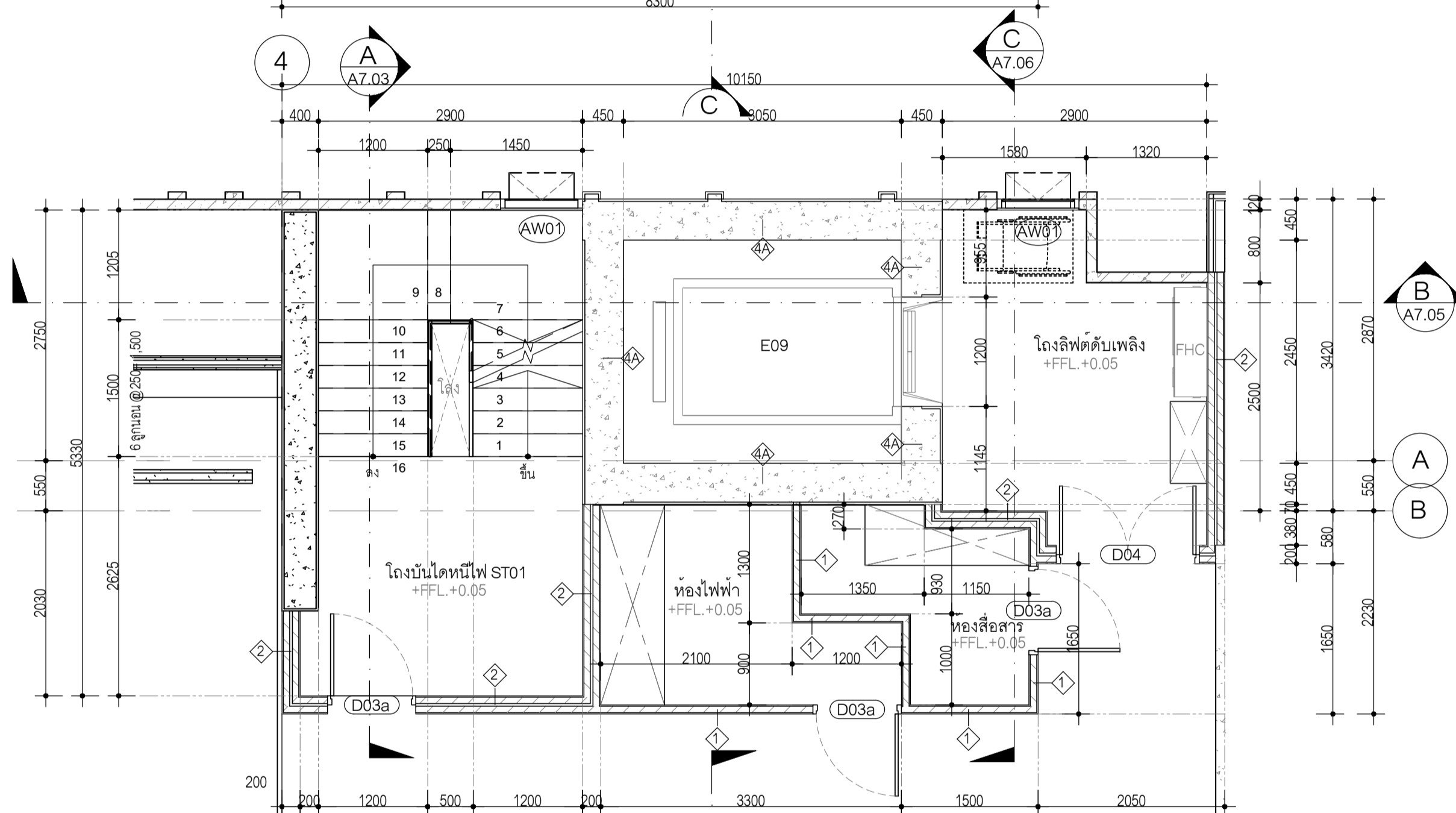
ผังพื้นที่ P3-P9
