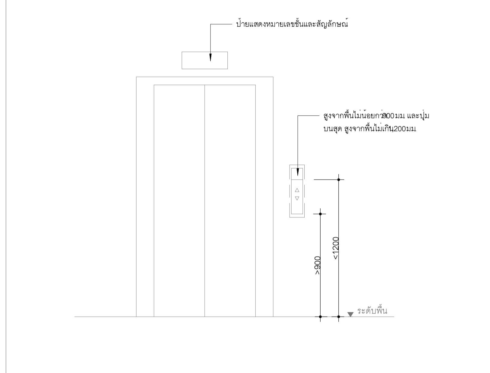
2 แบบขยายปุ่มกดหน้าลิฟต์ทั่วไป มาตรฐาน 1 : 20
