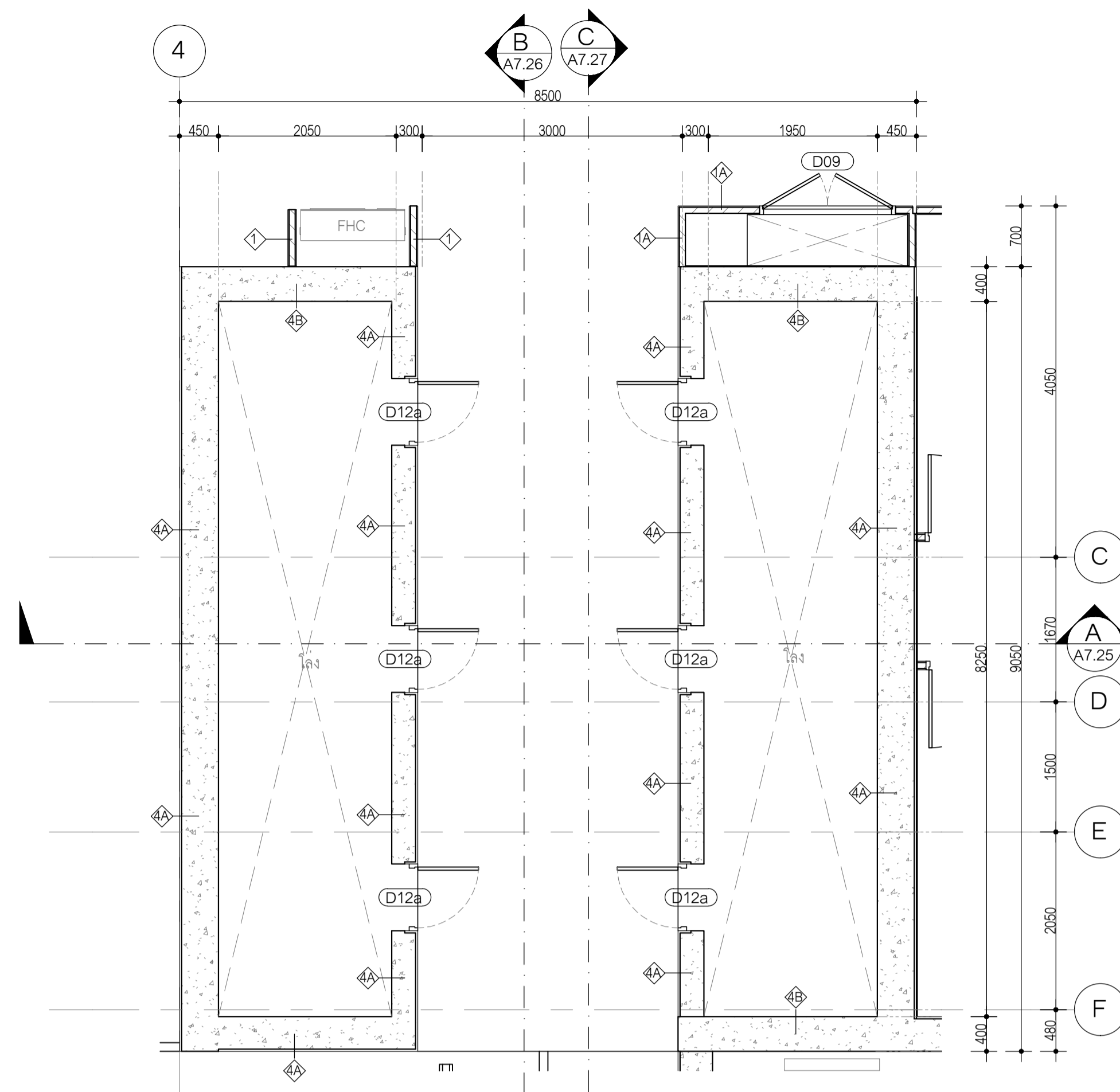
ผังพื้นที่ P4,P7,P10
