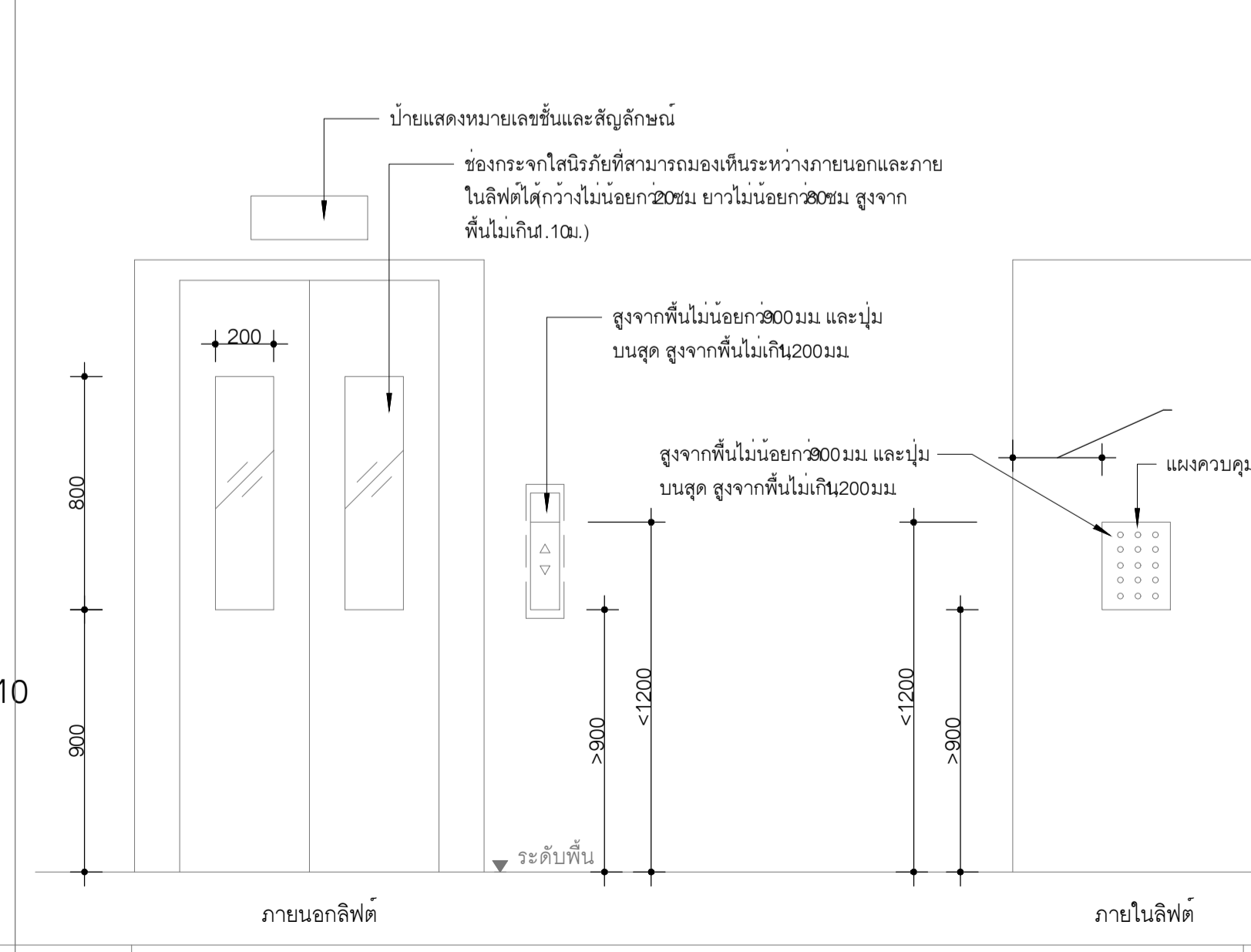
3 แบบขยายปุ่มกดหน้าลิฟต์ผู้พิการ มาตรฐาน 1 : 20
